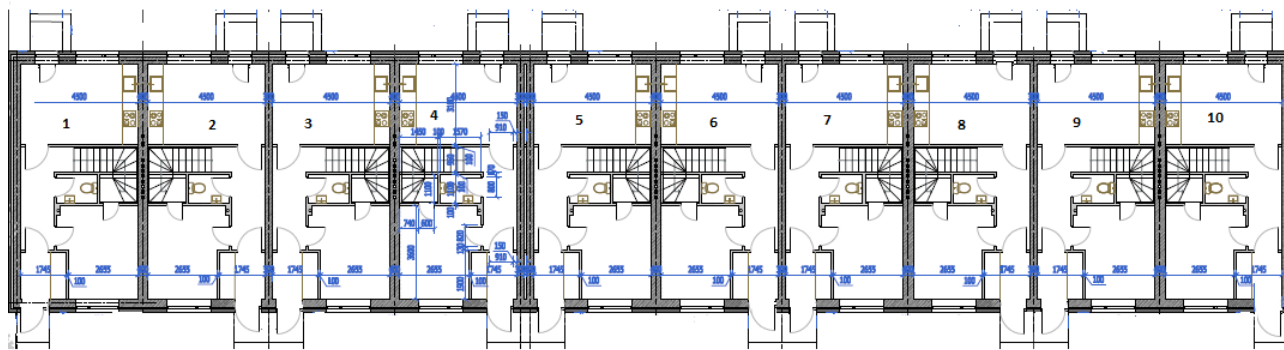
План 1 этажа
