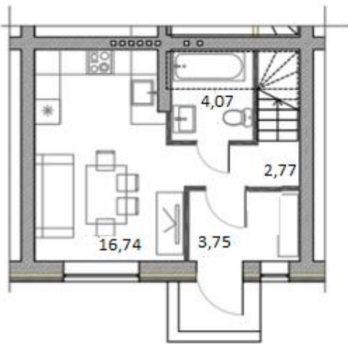
План 1 этажа
