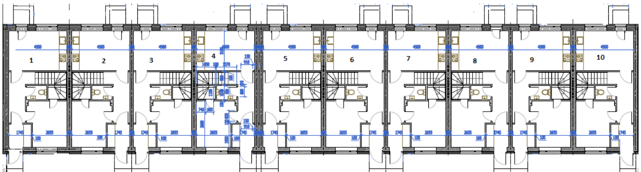
План 1 этажа
