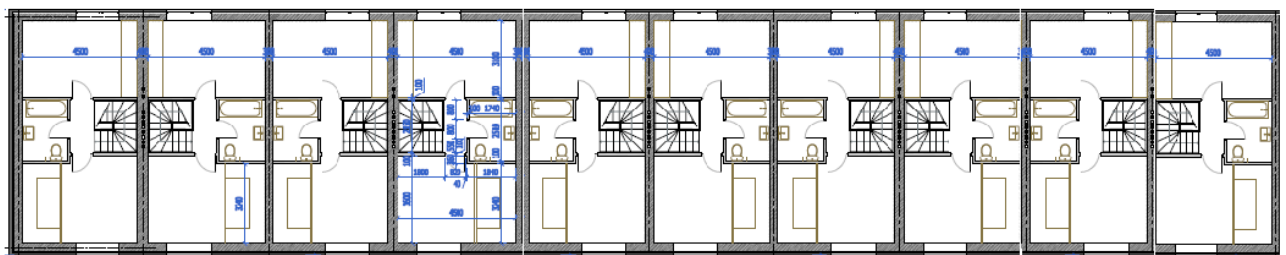
План 2 этажа
