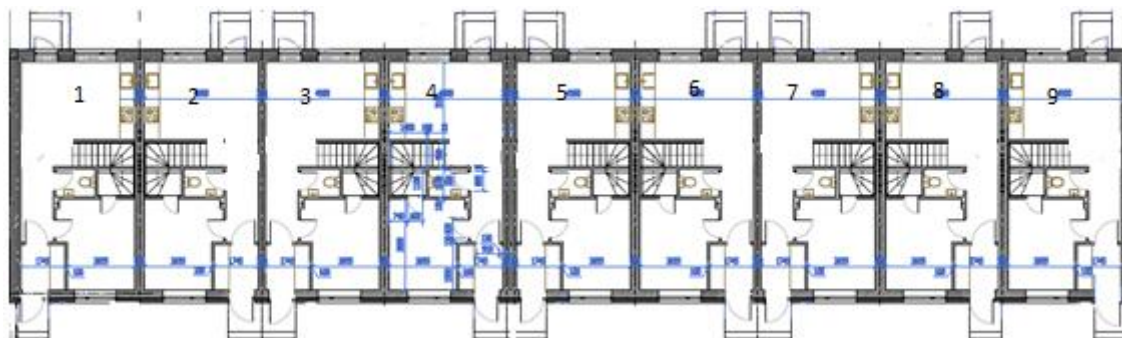
План 1 этажа
